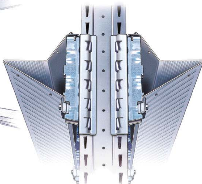
21 Profilo guida DRIVE-IN bifronte con staffa singola
