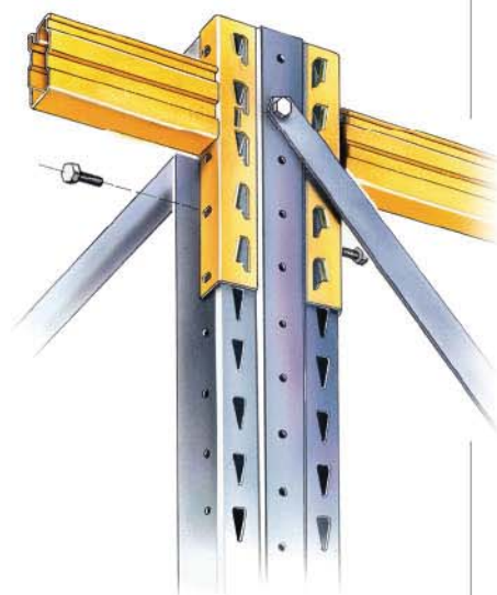
Ancoraggio in sommità (particolare dell'ancoraggio)
