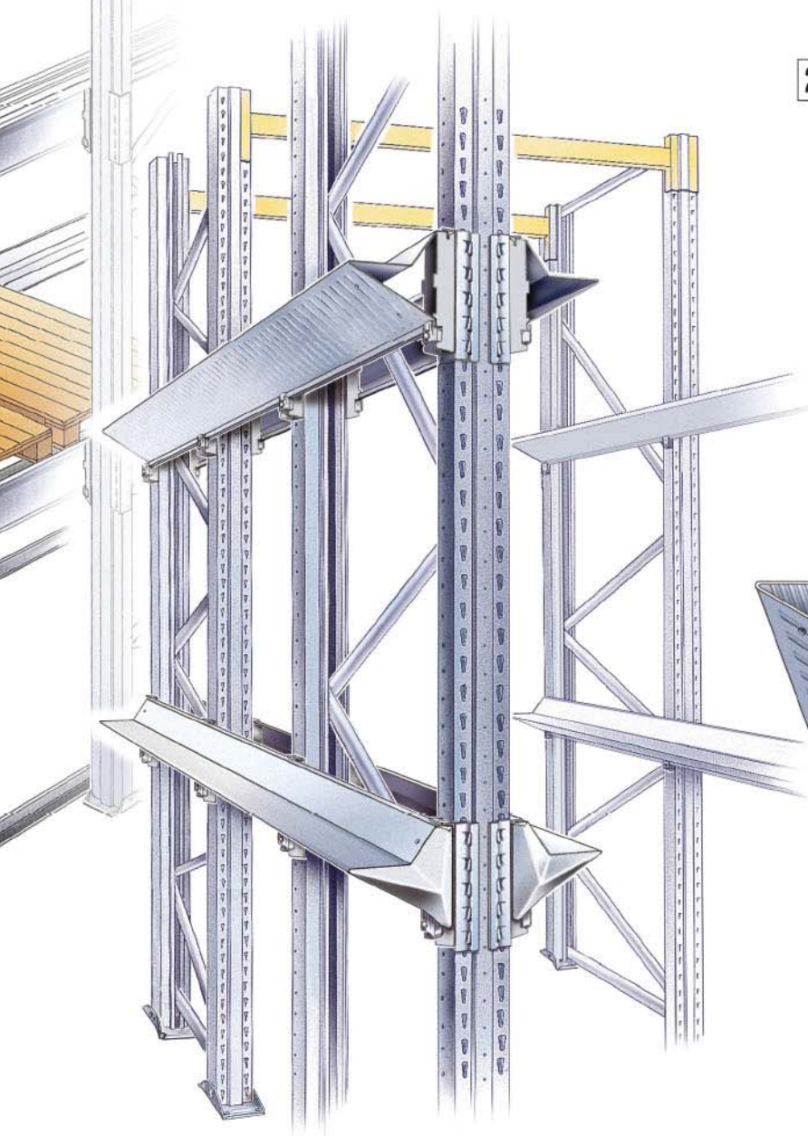
21 Profilo guida DRIVE-IN bifronte con staffa singola
